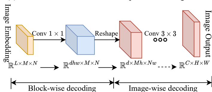
(d) CNeRV decoder
